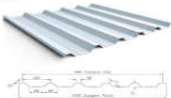
Figura 2 - Imagem telha metálica trapezoidal TP40-950
